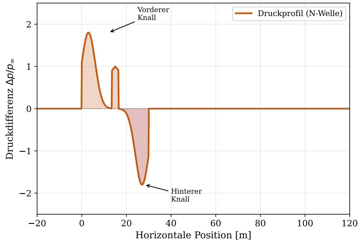
Konventionelles Überschallflugzeug (klassische N-Welle)
