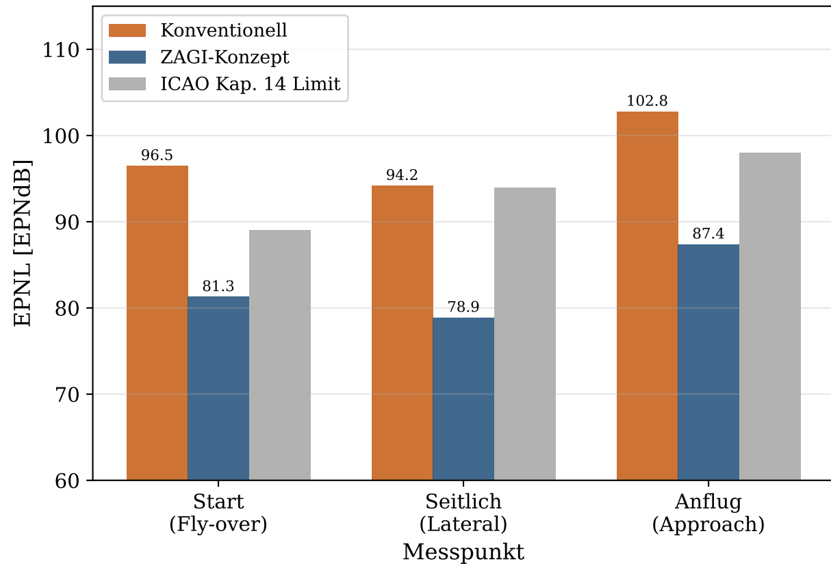
Effektiver wahrgenommener Lärmpegel (EPNL) nach ICAO Annex 16
