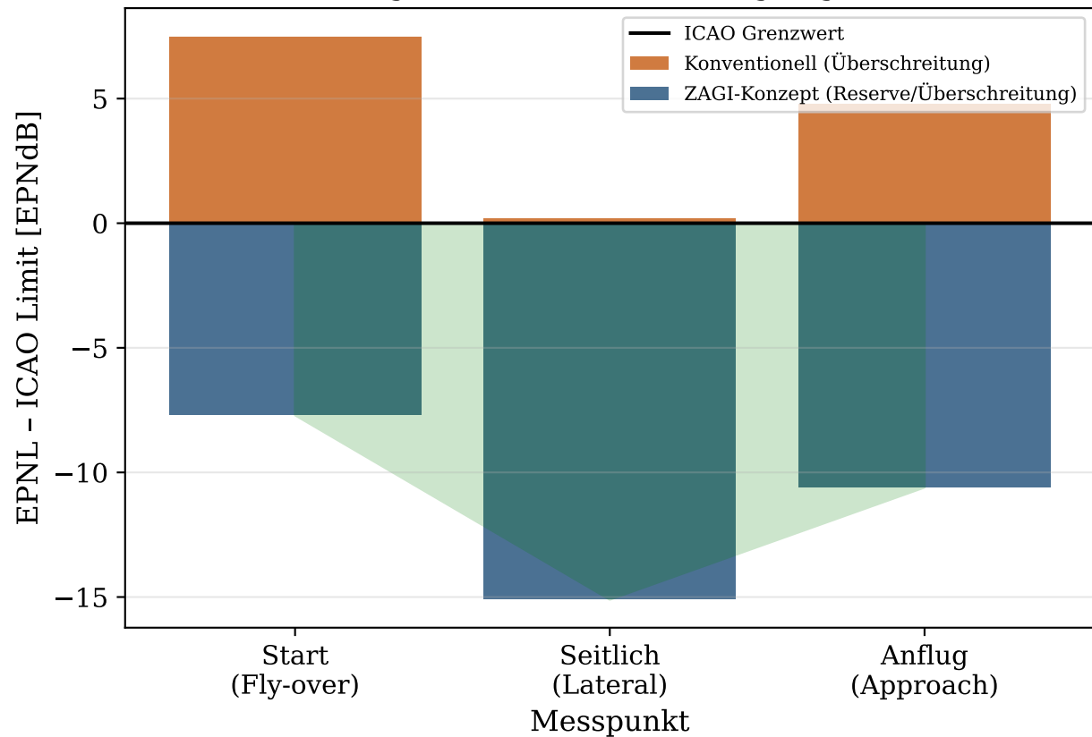
Lärmreserve relativ zum ICAO Kap. 14 Grenzwert (negativ = Unterschreitung = gut)
