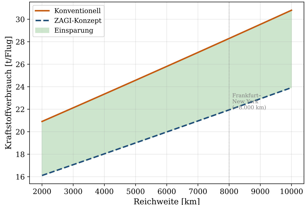
Kraftstoffverbrauch vs. Reichweite bei optimaler Reisemachzahl
