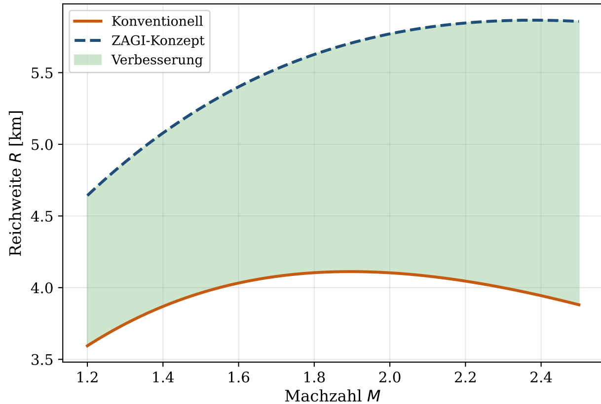
Theoretische Reichweite (Breguet-Gleichung) vs. Machzahl
