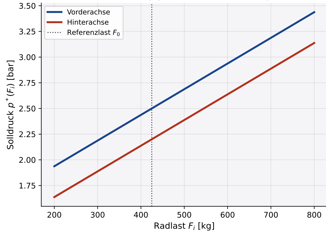
Lastabhängige Solldruck-Skalierung
