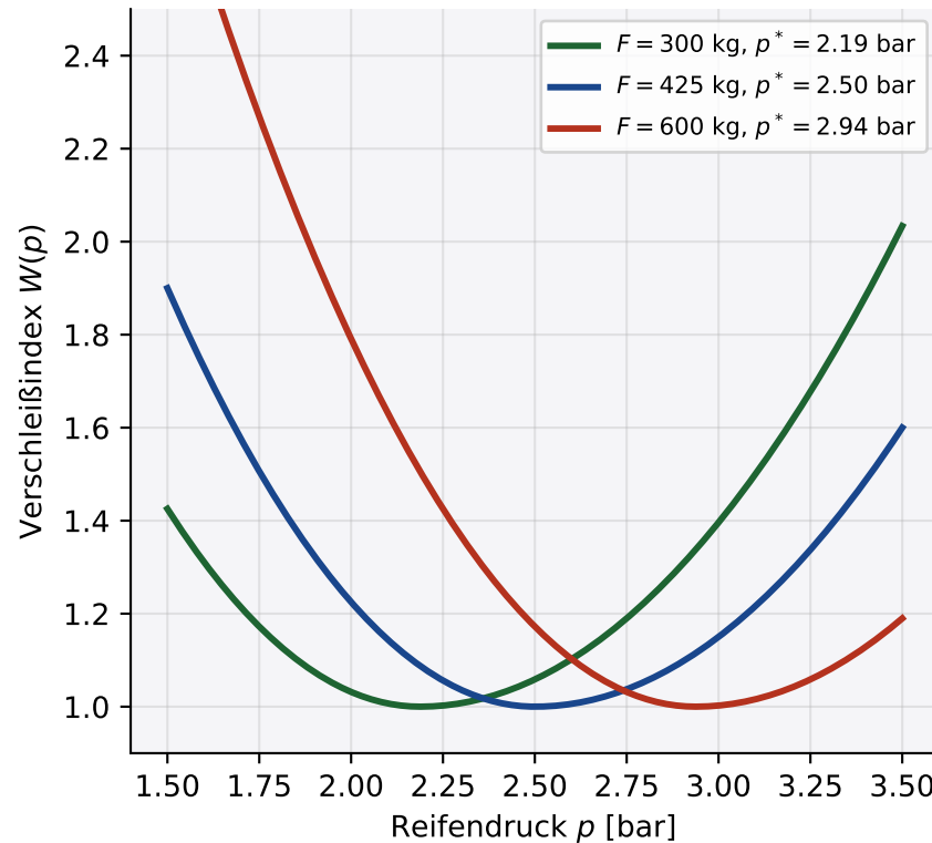
Lastabhängiger Verschleißindex
