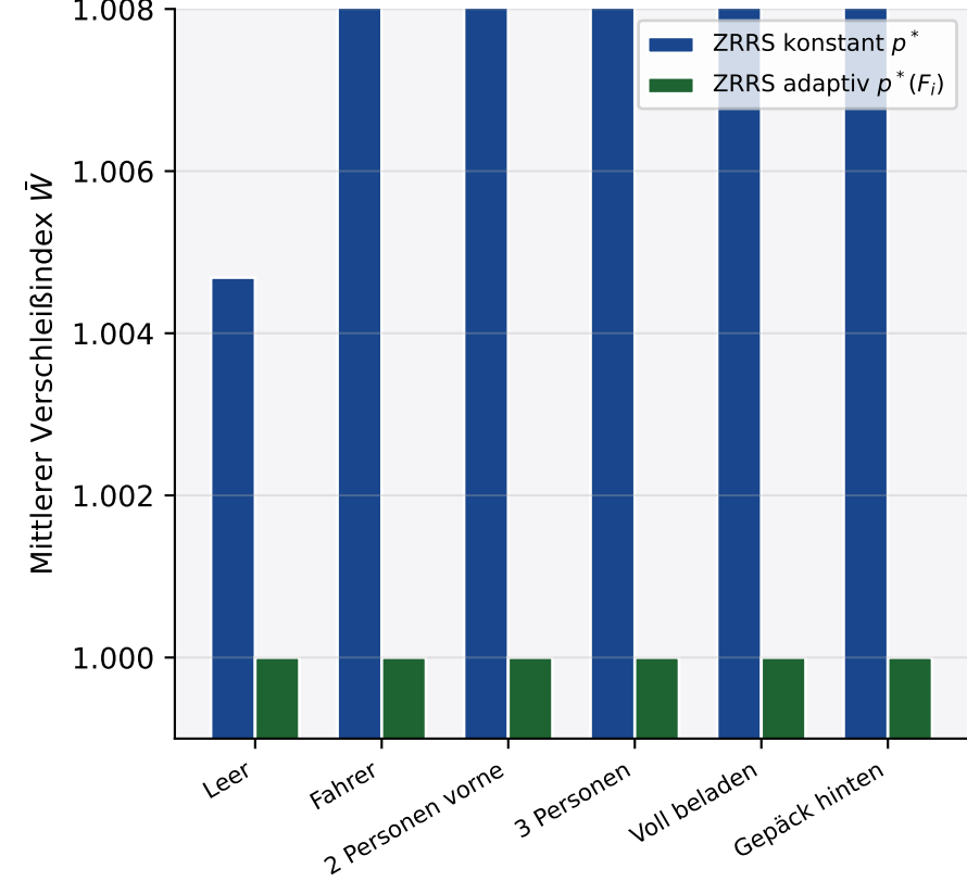
Konstant vs. adaptiv bei Beladungsszenarien
