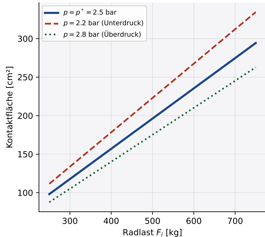
Reifenkontaktfläche
