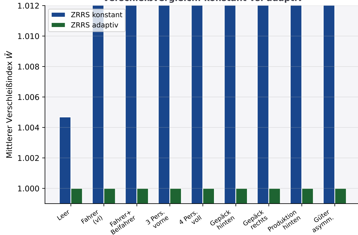
Verschleißvergleich: konstant vs. adaptiv
