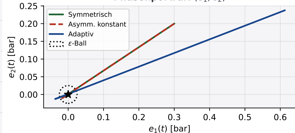
Phasenportrait ( e_1, e_2 )
