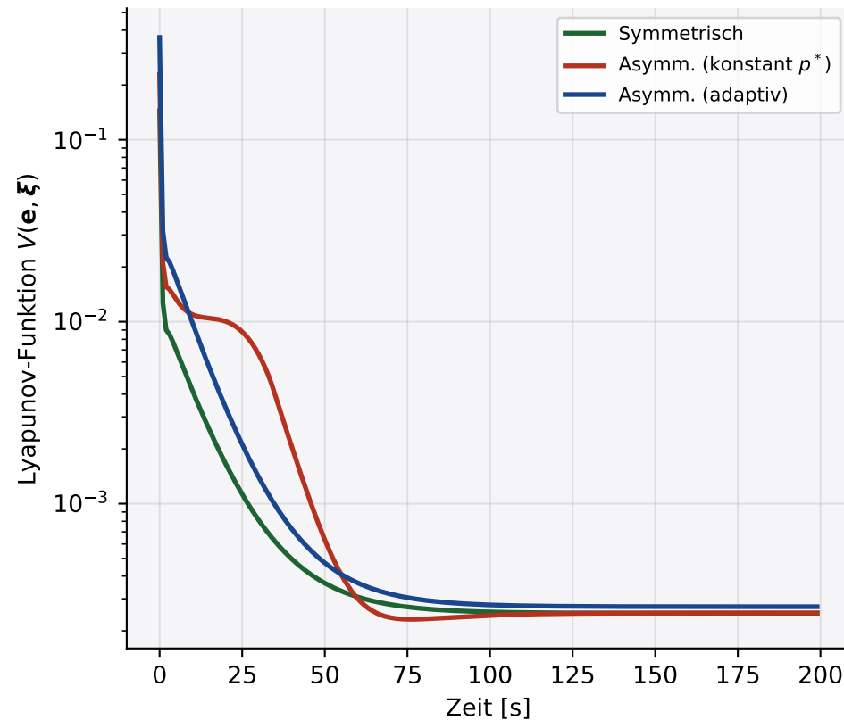
Lyapunov-Abfall (logarithmisch)
