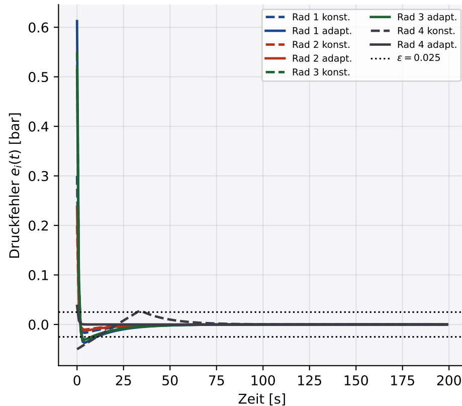
Fehlerentwicklung je Rad
