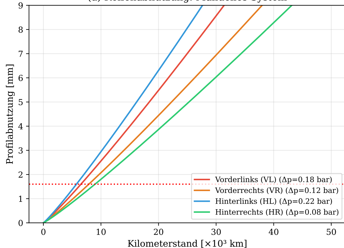
(a) Reifenabnutzung: Manuelles System
