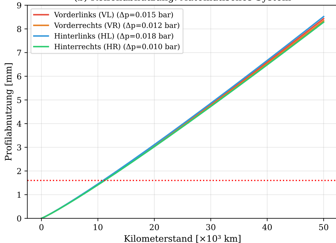
(b) Reifenabnutzung: Automatisches System
