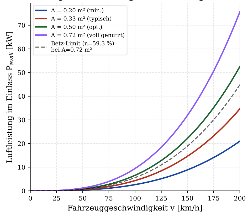
Verfügbare Luftenergie im Fahrzeugeinlass
