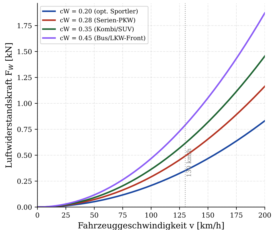
Luftwiderstandskraft
