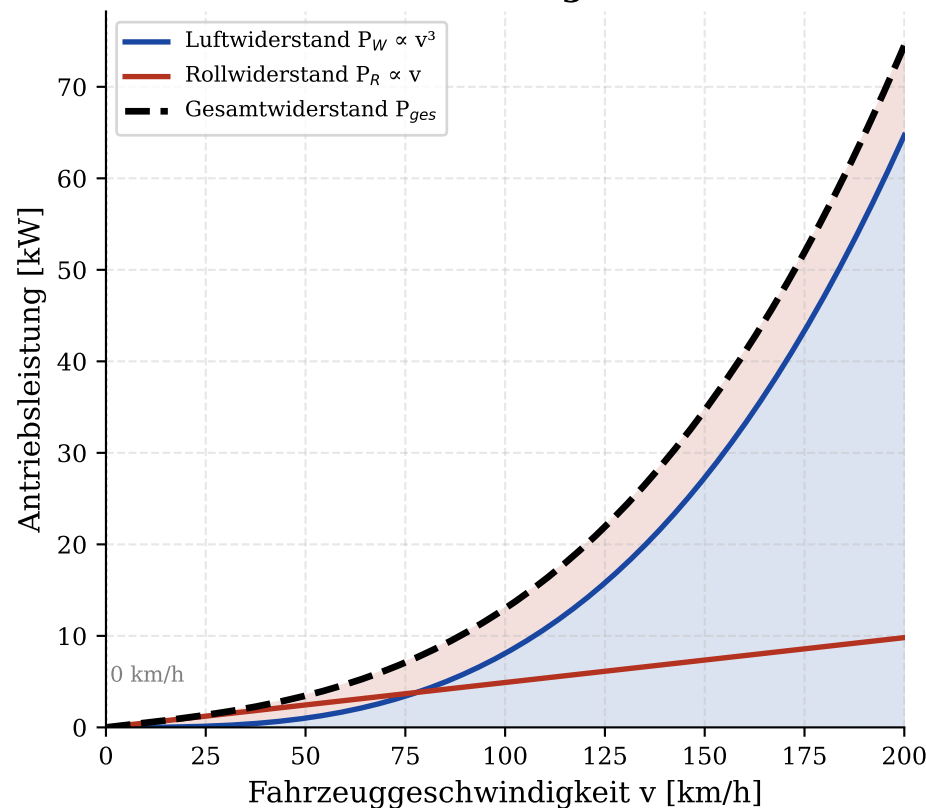
Antriebsleistungsanteile
