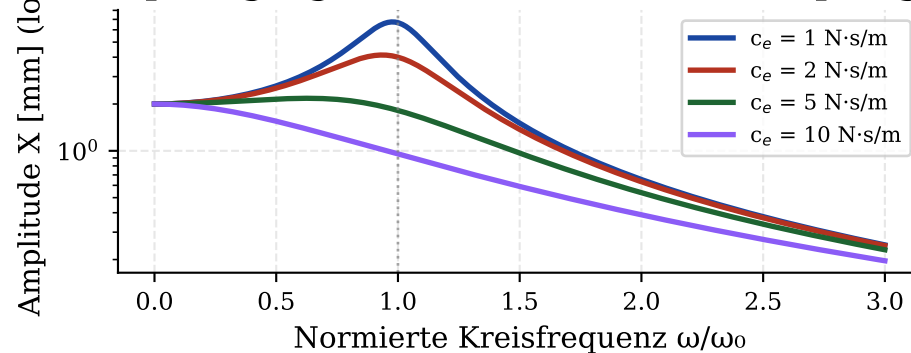
Frequenzgang bei verschiedenen el. Dämpfungen
