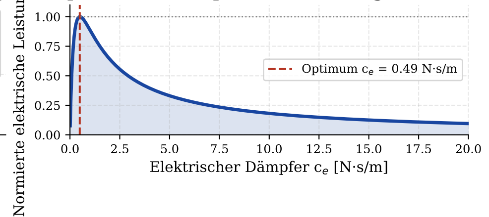
Optimaler Arbeitspunkt der Leistungsextraktion
