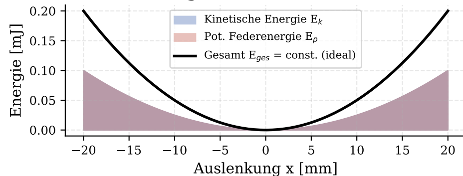
Energiebilanz Feder-Masse
