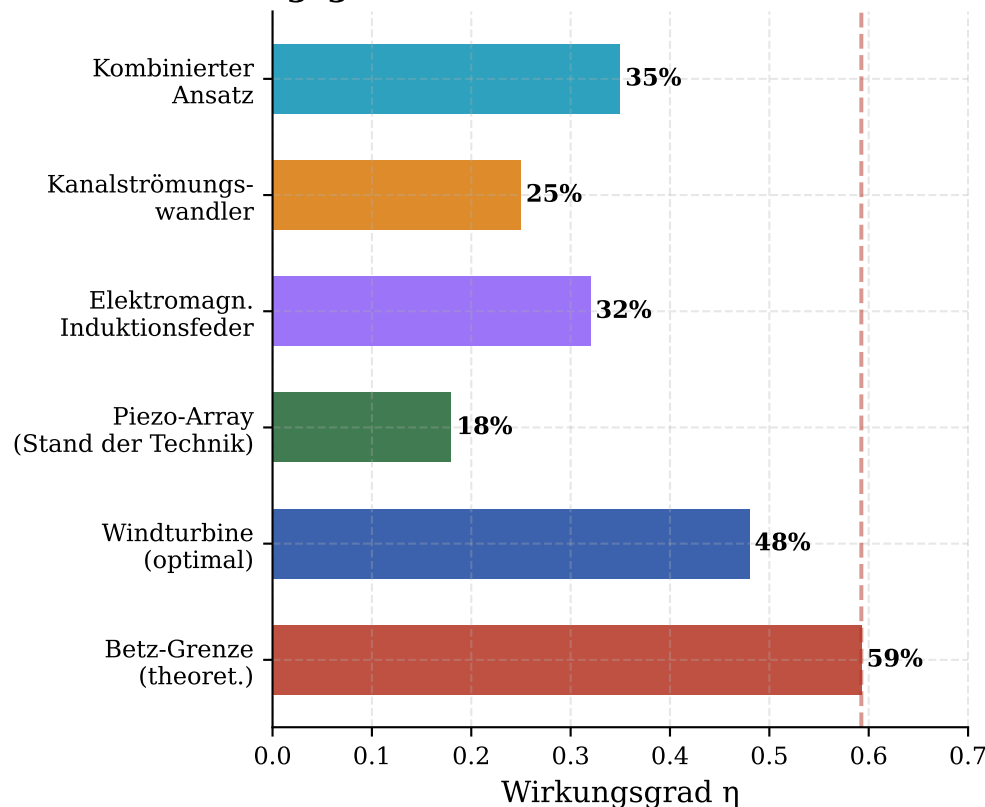
Wirkungsgrade verschiedener Wandlertechnologien
