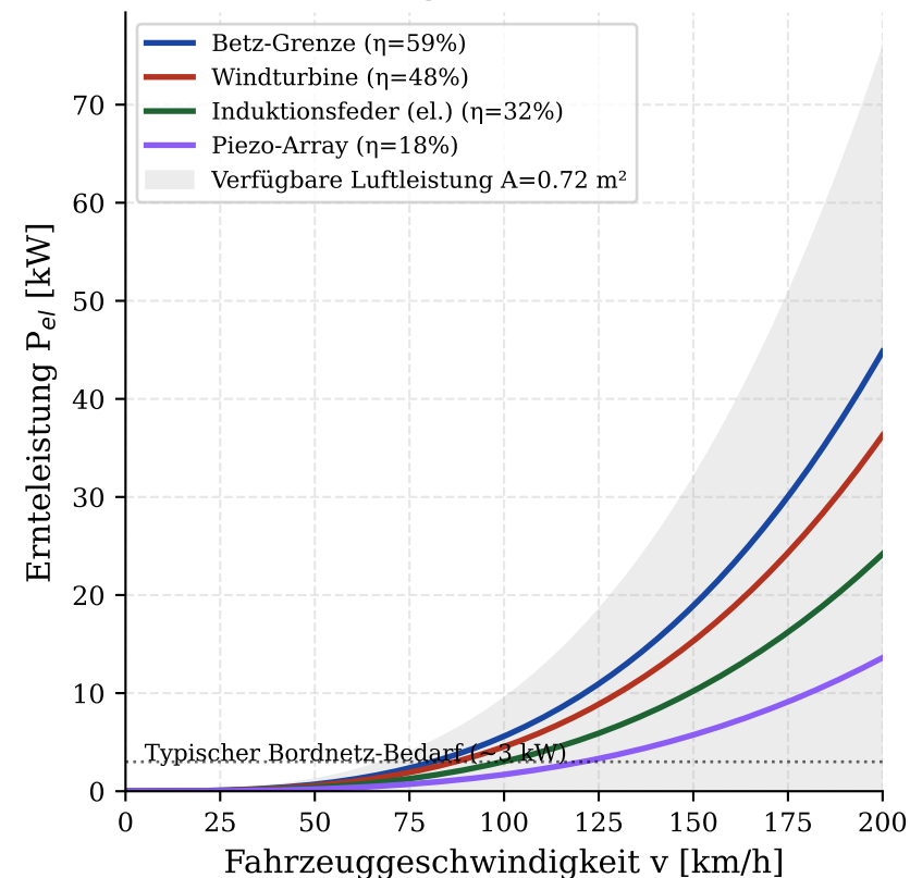
Ernteleistung bei A_{\text{intake}} = 0.72 \text{ m}^2
