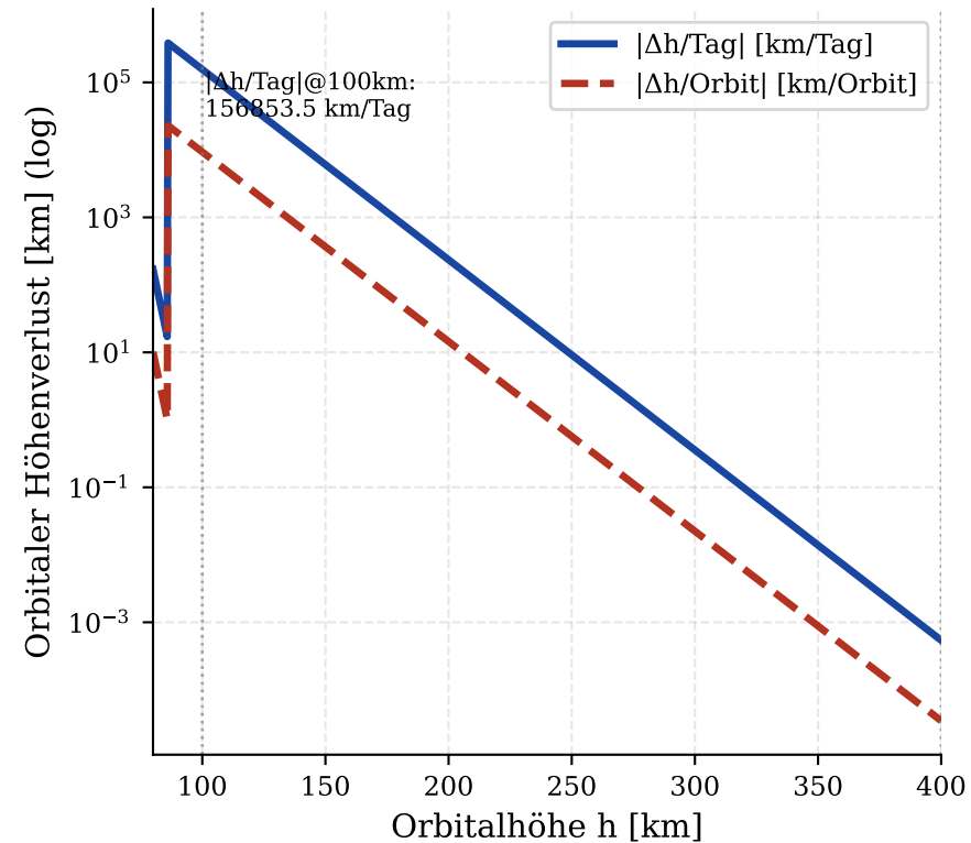
Orbitaler Höhenverlust durch atmosph. Abbremsung
