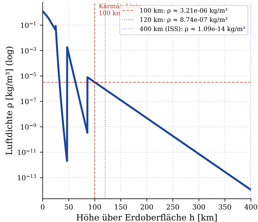
US-Standardatmosphäre: Dichteprofil
