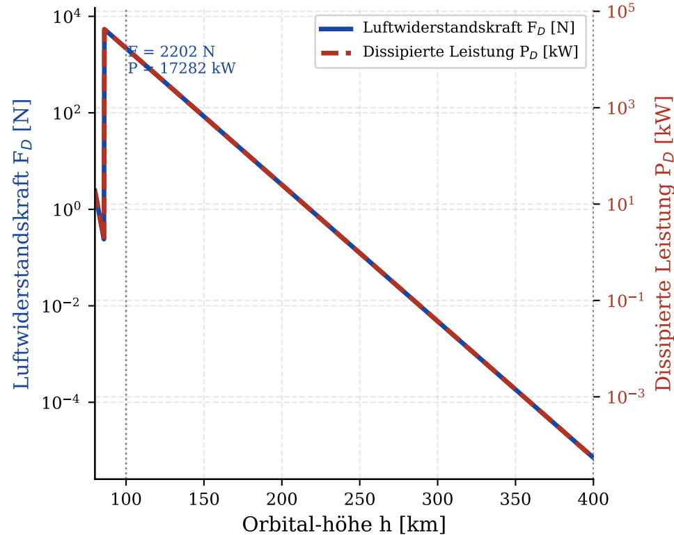
Luftwiderstand auf Satelliten ( m=1000.0 kg, A=10.0 m 2 , C_D=2.2 )
