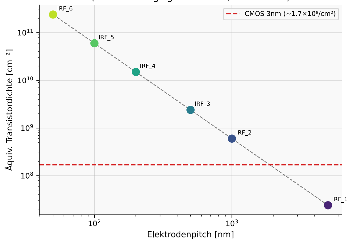
IRF Transistordichte vs. Pitch (alle Technologiegenerationen, 3 Schichten)
