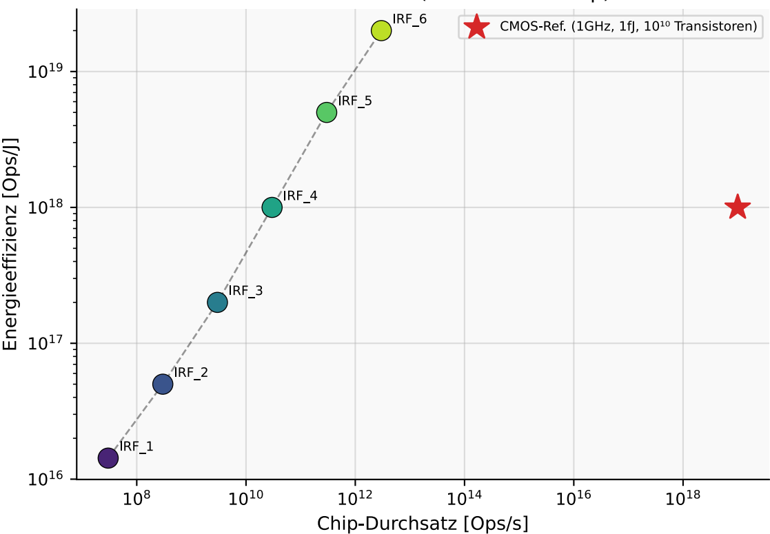
Energieeffizienz-Karte IRF-Generationen (100×100×3 Chip)
