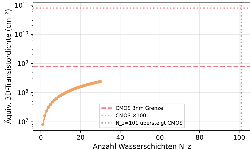
3D-IRF-Skalierung: \rho_{3D} = N_z \cdot 2 \cdot \rho_{2D} ( p=5 \mu\text{m} )
