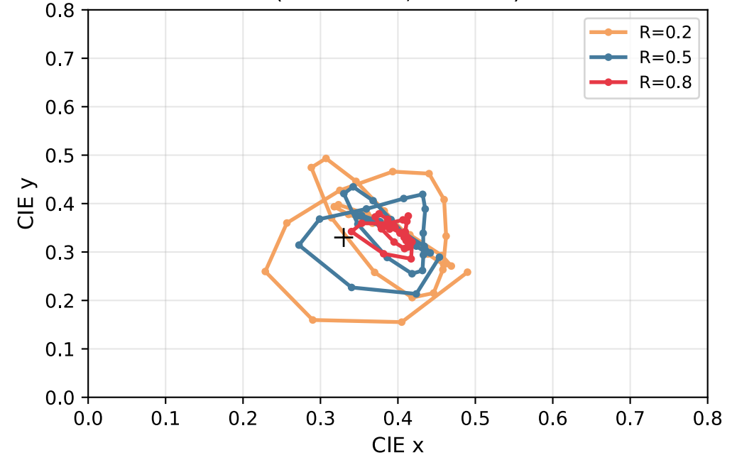
CIE-Farbgamut vs. Quellungsgrad Q ( d_0=250\text{nm} , n_0=1.50 )
