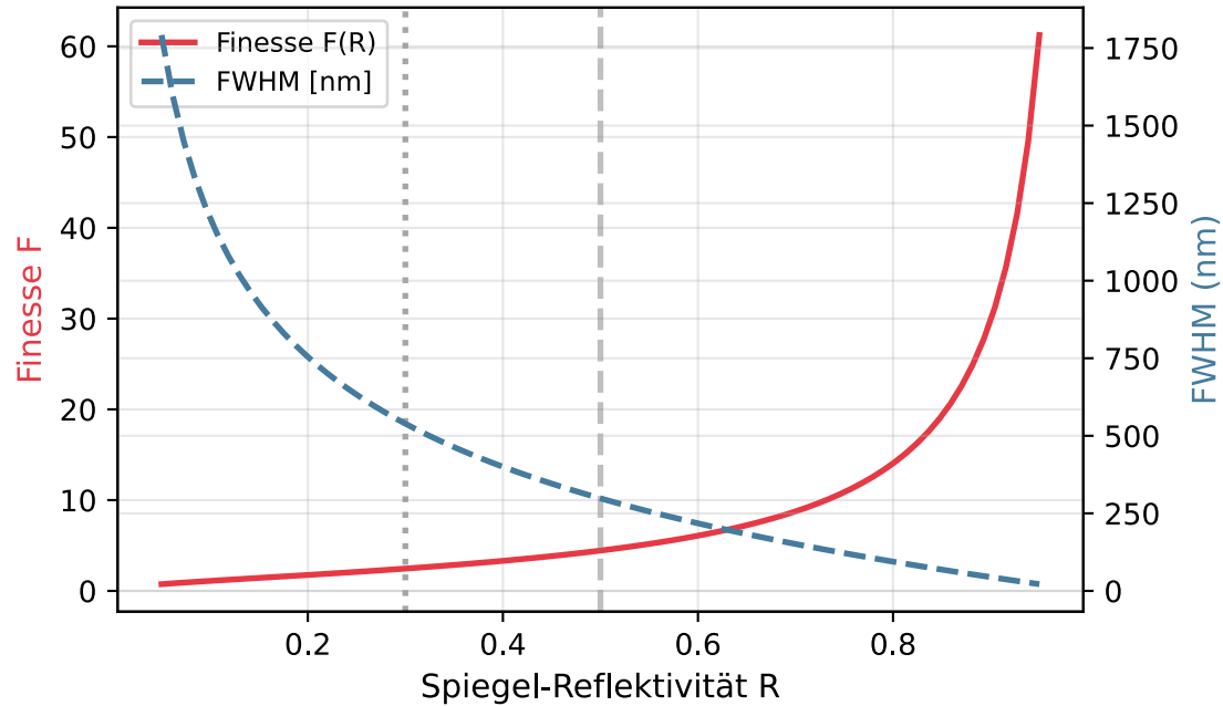
Finesse und FWHM als Funktion von R ( d_0=250\text{nm} , Q=2.15 )
