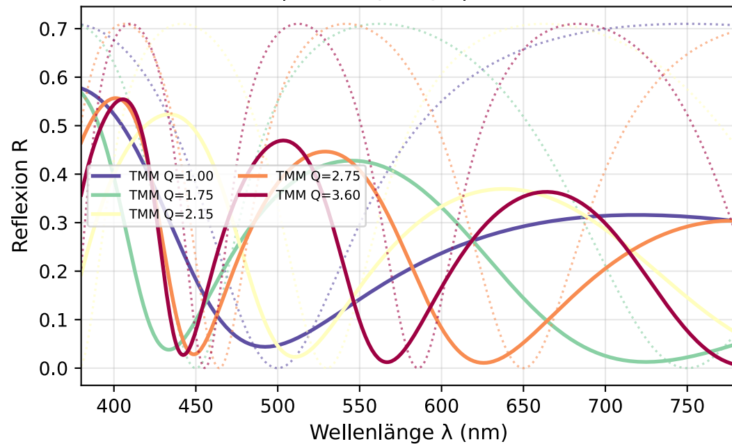
TMM (durchgehend) vs. FP-Modell (gepunktet) Au|PDMS-Hydrogel|Au Stack
