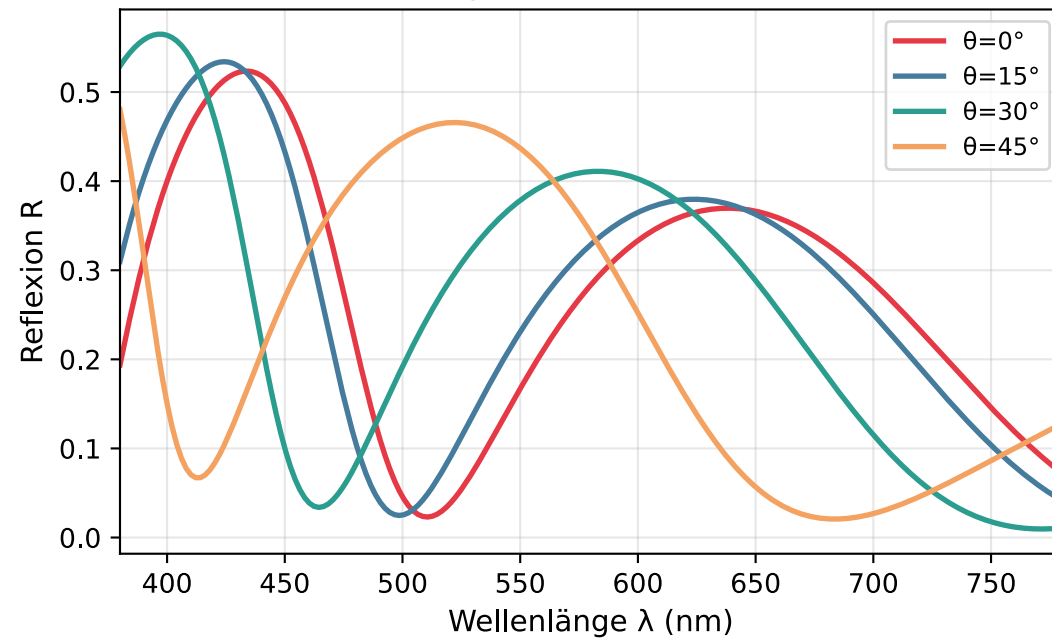
Winkelabhängigkeit R(\lambda, \theta) bei Q=2.15 (unpolarisiertes Licht)
