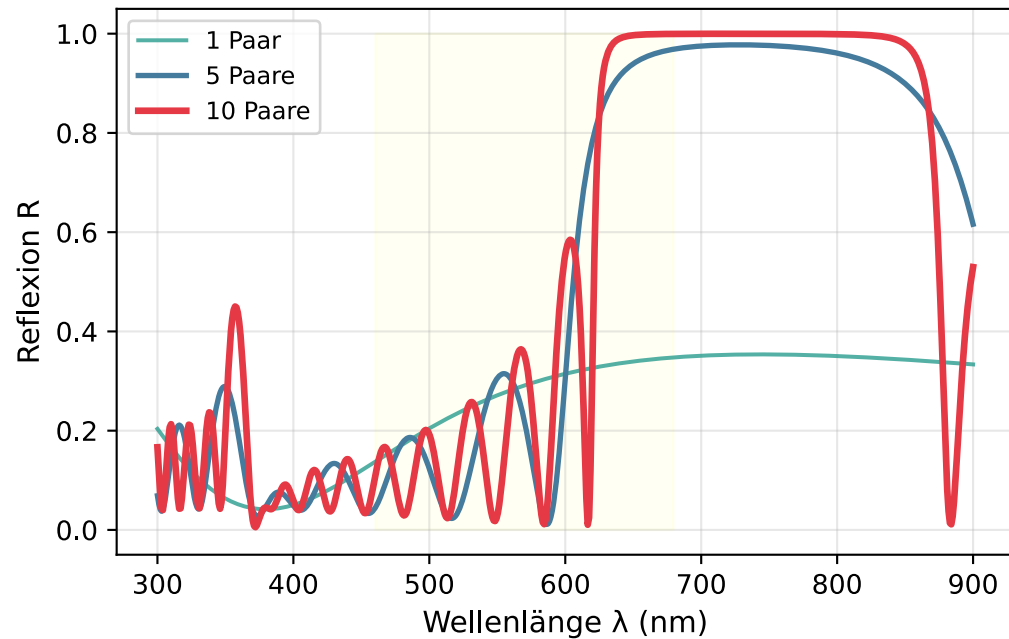
Photonischer Kristall: \text{TiO}_2/\text{SiO}_2 -Bragg-Spiegel Bandlücke wächst mit Schichtzahl
