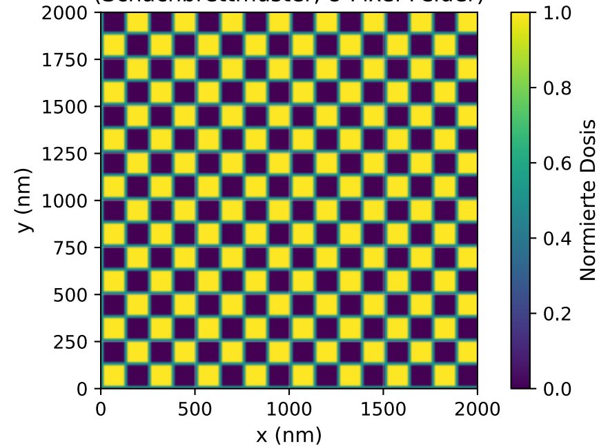
Proximity-korrigiertes Belichtungsmuster (Schachbrettmuster, 8-Pixel-Felder)
