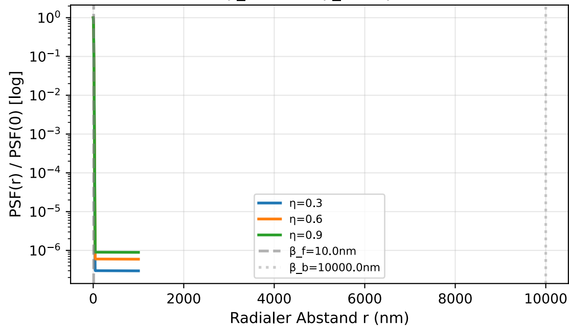
Chang-Doppel-Gauss-PSF für verschiedene \eta -Werte ( \beta_f=10\text{nm} , \beta_b=10\mu\text{m} )
