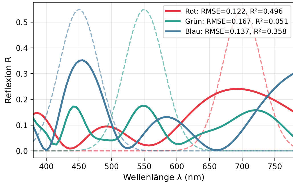
RGB-Primärfarben: Ziel (—) vs. optimiert (--) Adjungierter Gradientenabstieg
