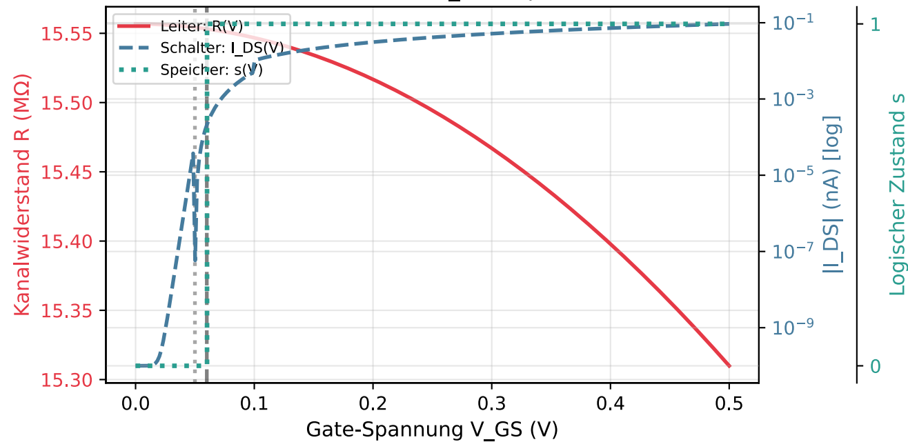
Dreifache Simultaneität: Leiter (R), Schalter ( I_{DS} ), Speicher (s)
