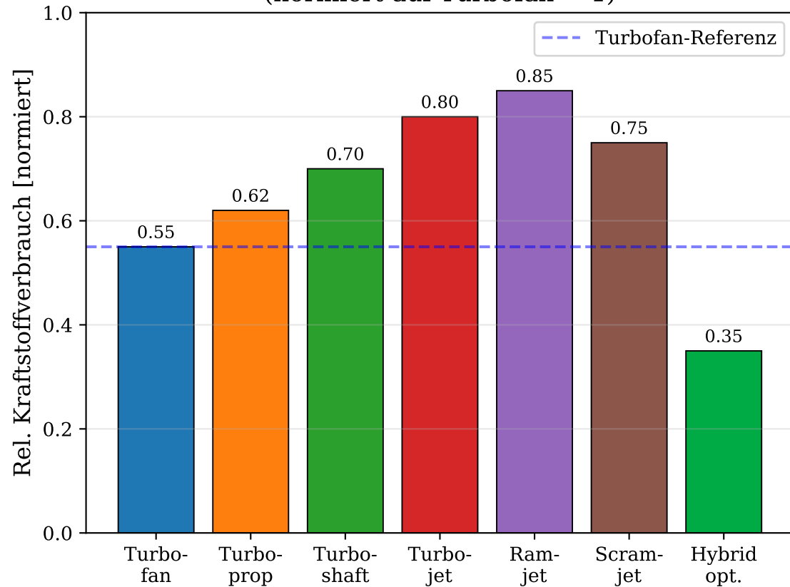
Kraftstoffverbrauch im Reiseflug (normiert auf Turbofan = 1)
