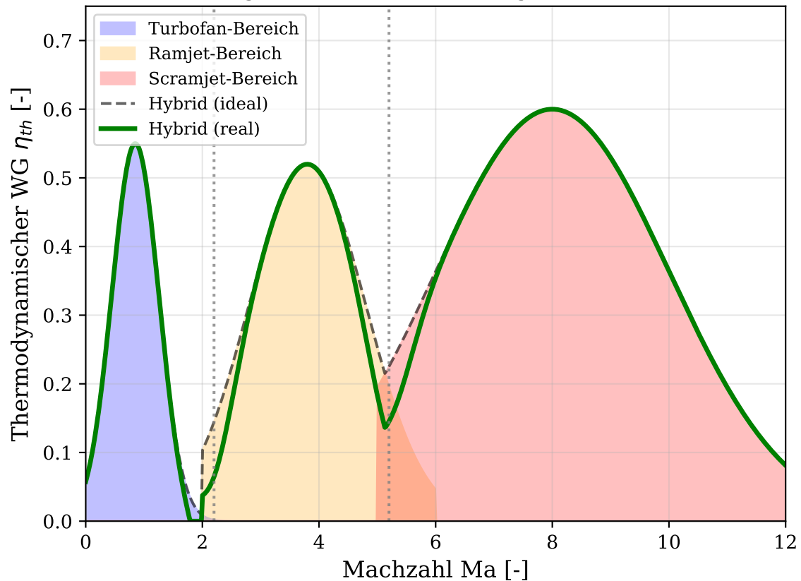
Hybridtriebwerk: Wirkungsgrad über den gesamten Geschwindigkeitsbereich
