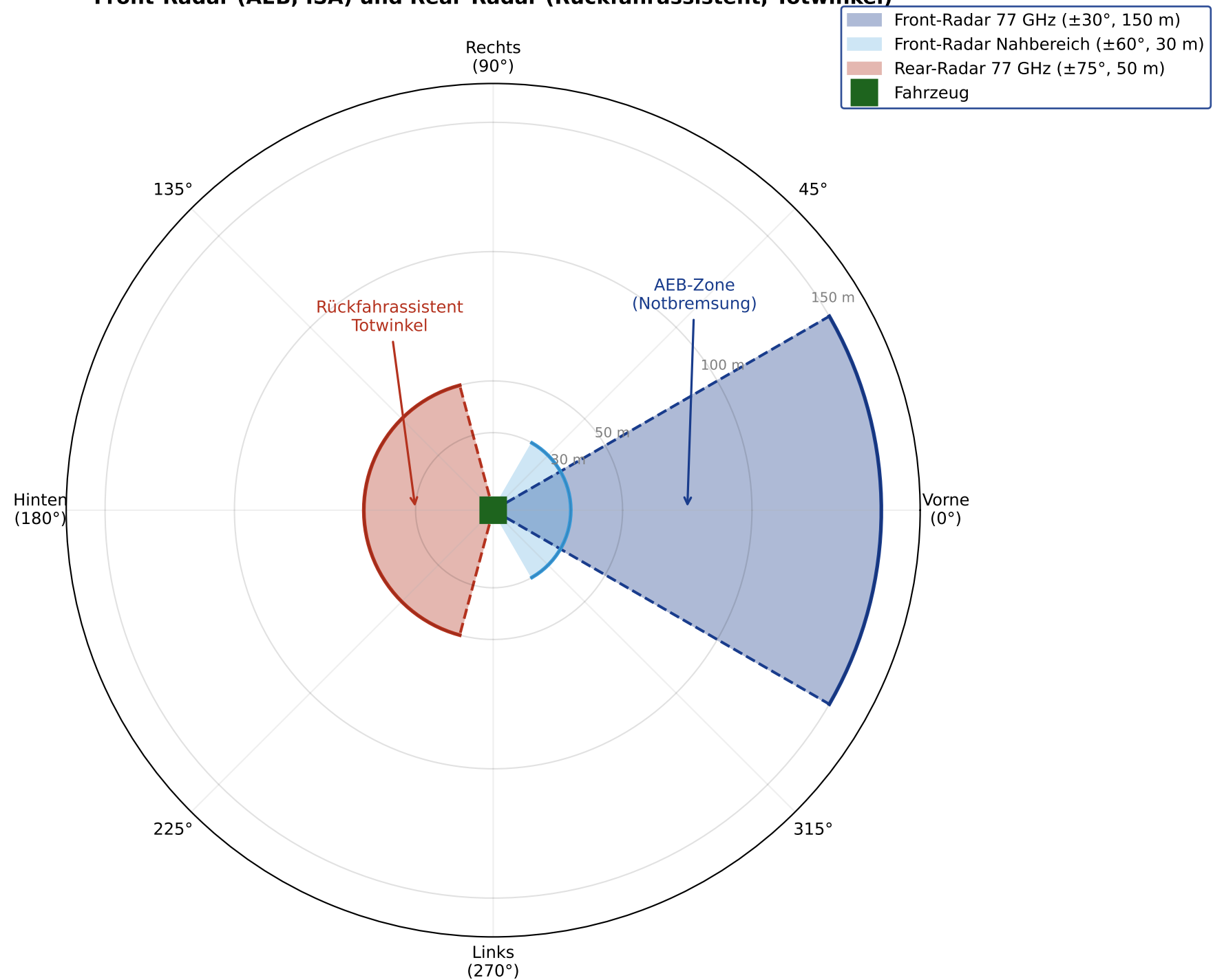
Abbildung 1: Radarabdeckung des Zwei-Sensor-Systems Front-Radar (AEB, ISA) und Rear-Radar (Rückfahrsassistent, Totwinkel)
