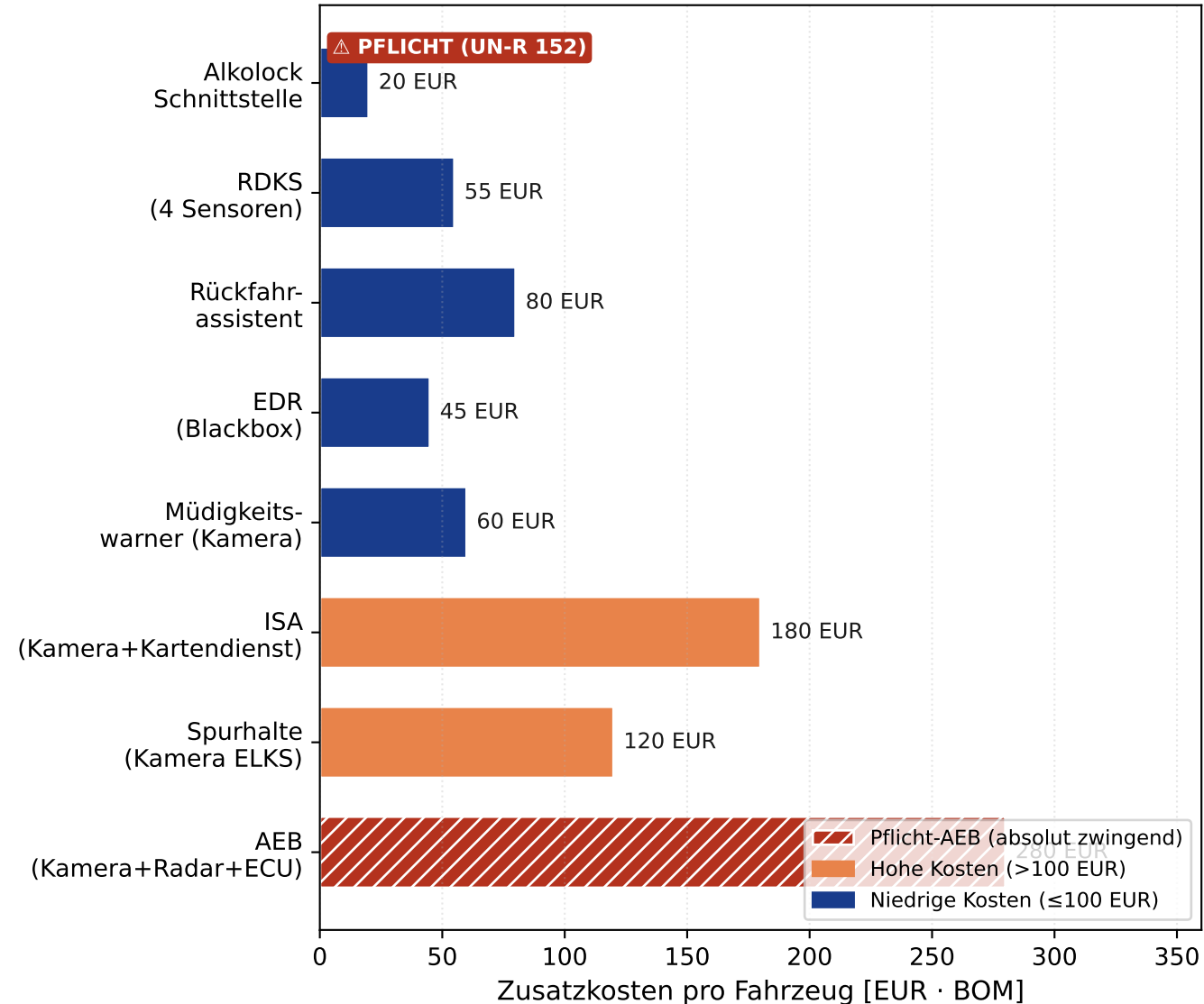
(a) Vollausstattung EU 2019/2144 Gesamtkosten: 840 EUR
