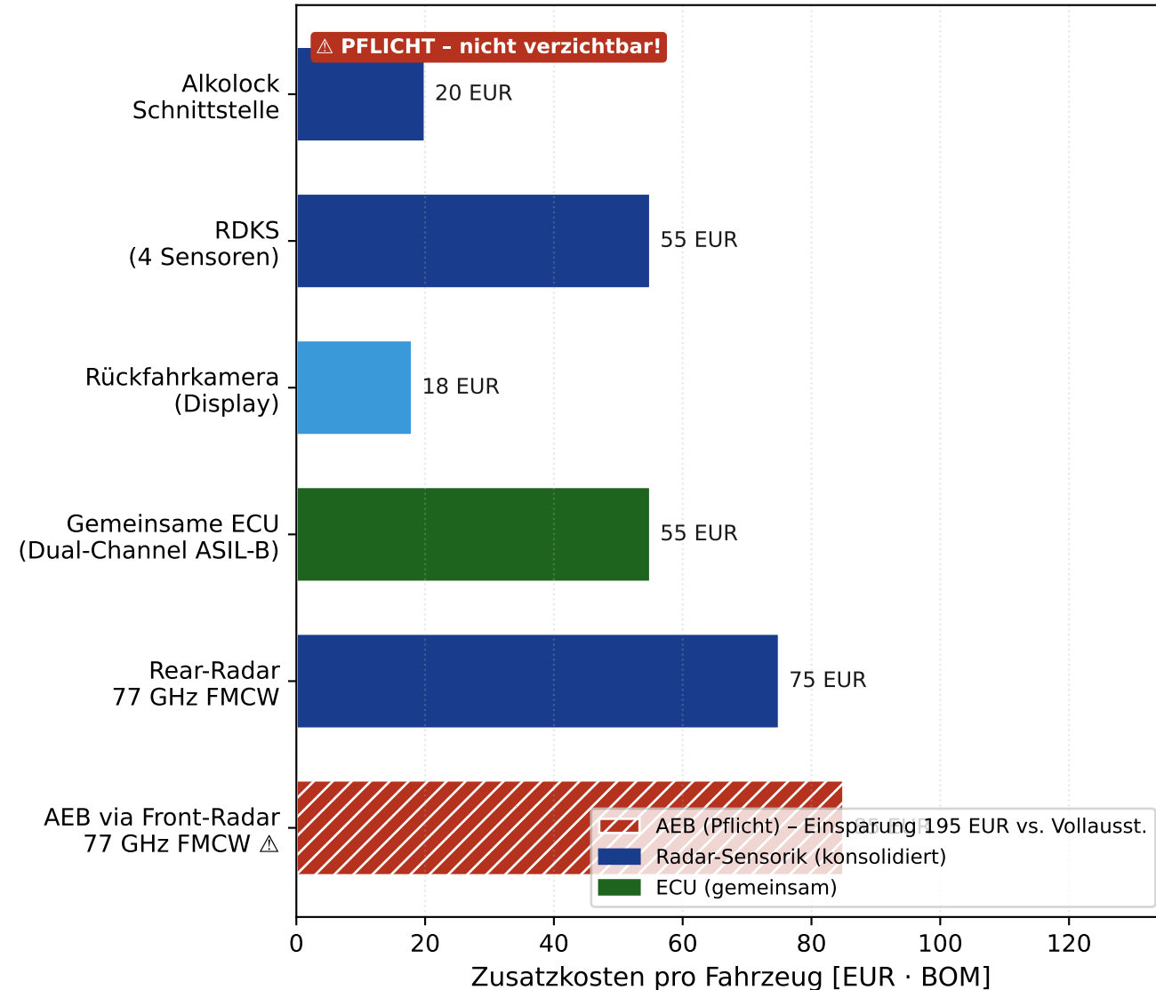
(b) Minimalsystem: AEB-Radar konsolidiert Gesamtkosten: 308 EUR
