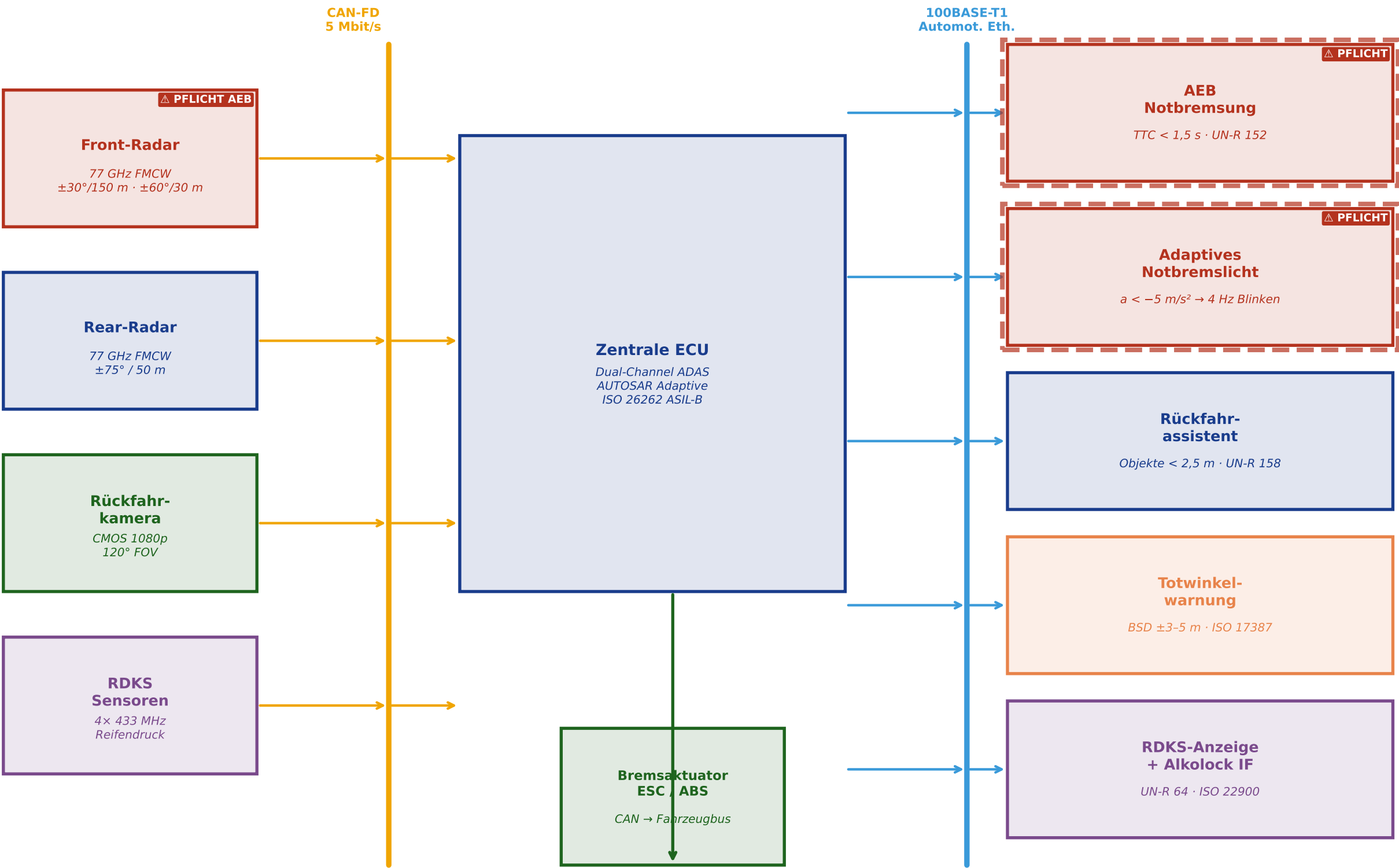
Abbildung 5: Systemarchitektur - AEB als zwingend vorgeschriebene Pflichtfunktion (Front-Radar realisiert AEB, Notbremslicht und Radardetektion auf einer Hardware)
