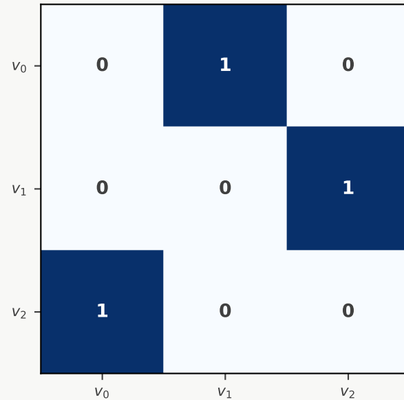
M_1 (3-Zykel)
