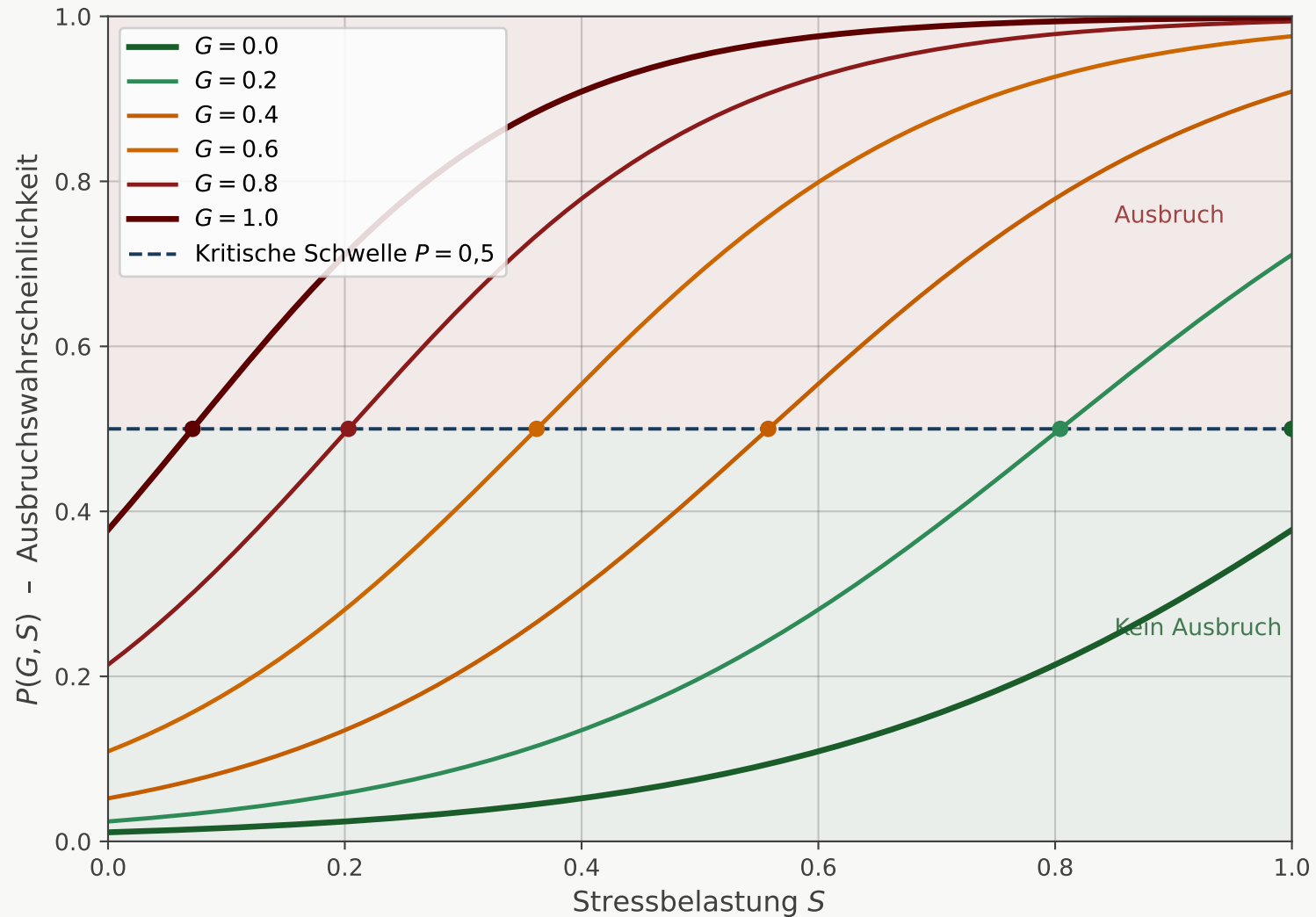
Querschnitte P(G_0, S) für feste Prädispositionswerte G_0
