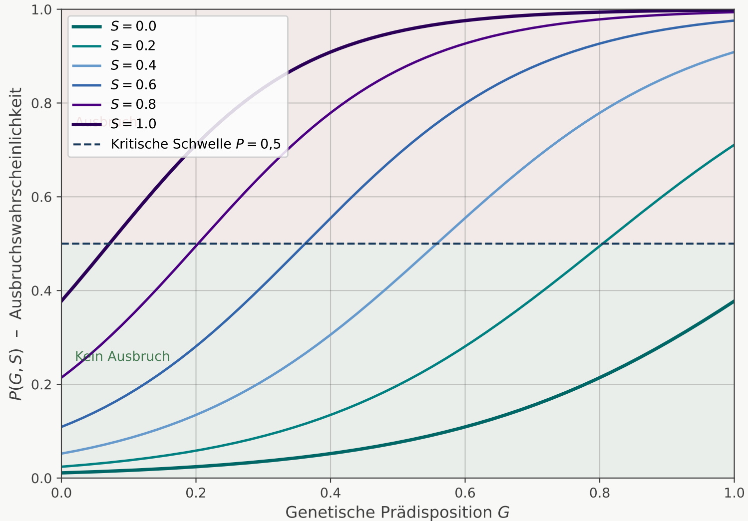
Querschnitte P(G, S_0) für feste Stressbelastungswerte S_0
