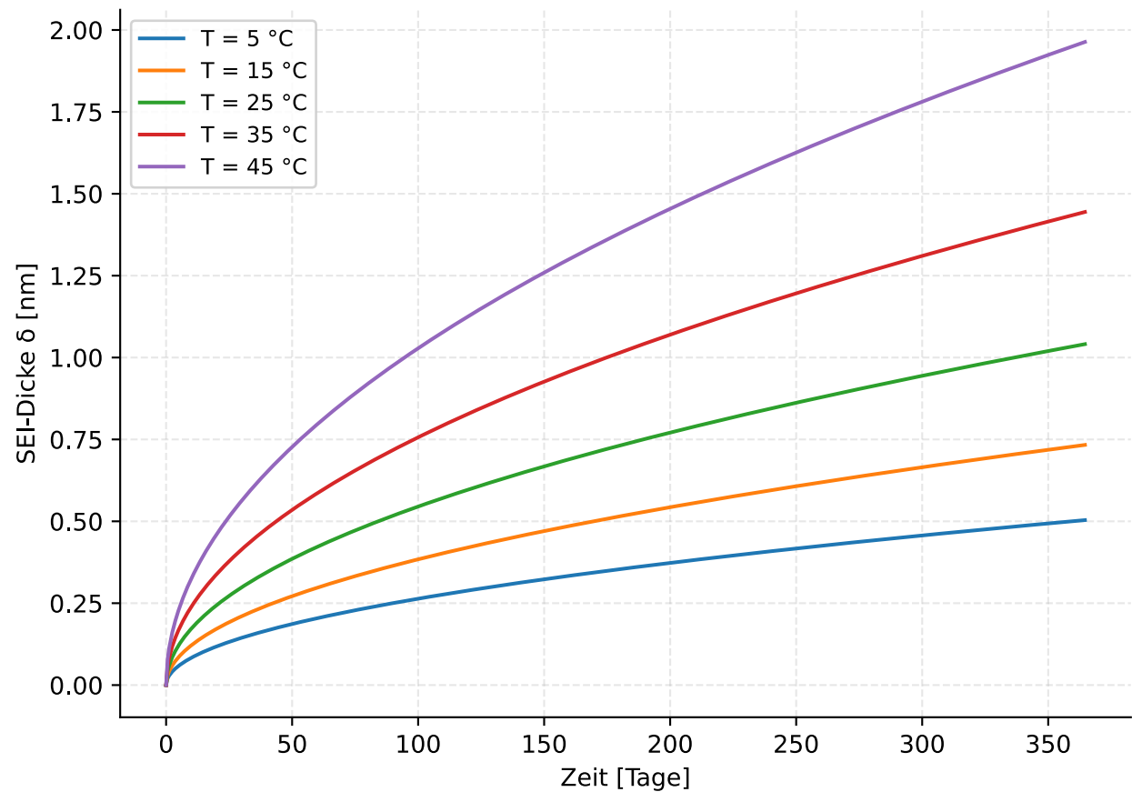
SEI-Schichtdickenwachstum \delta(t)
