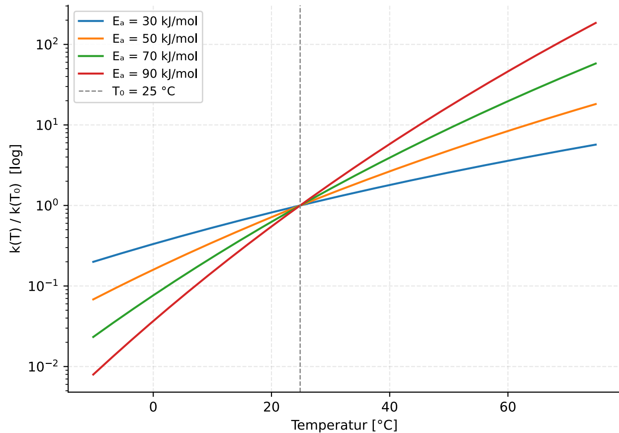
Arrhenius-Ratenverhältnis k(T)/k(T_0)
