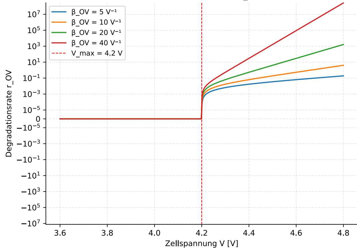
Überspannungsdegradation ( V_{\text{max}} = 4.2 \text{ V} )
