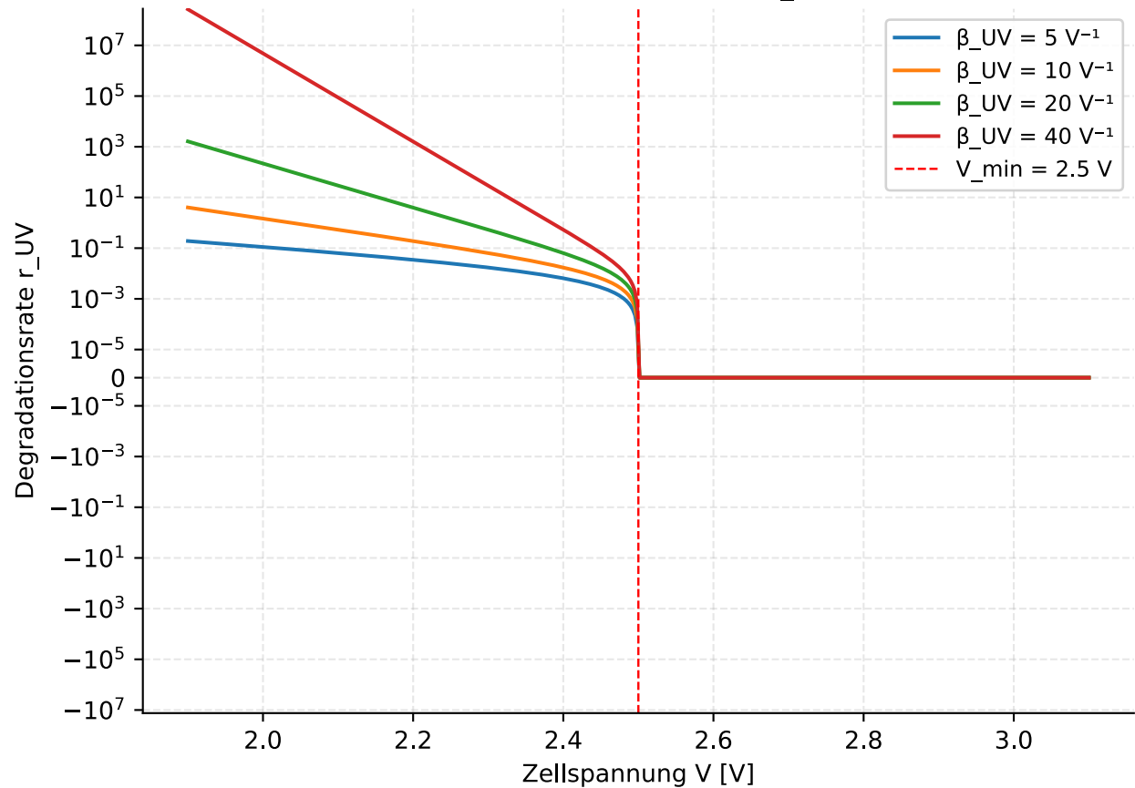
Unterspannungsdegradation ( V_{\text{min}} = 2.5 \text{ V} )
