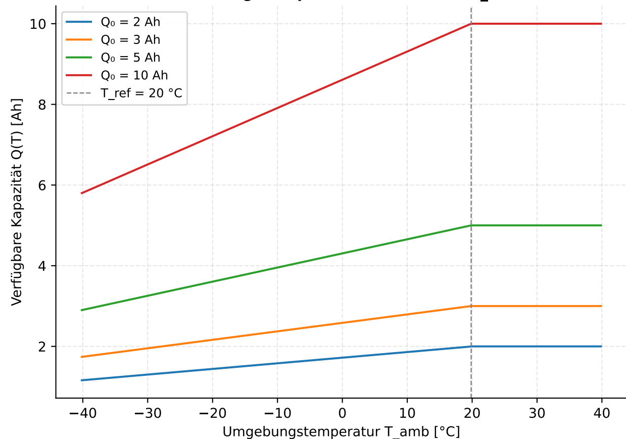
Kältebedingte Kapazitätsreduktion Q(T_{\text{amb}})
