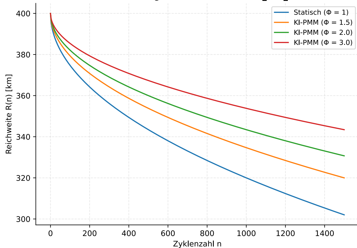
Reichweitenentwicklung R(n) ( R_0 = 400 km, n_{\text{EoL\_base}} = 1000 )
