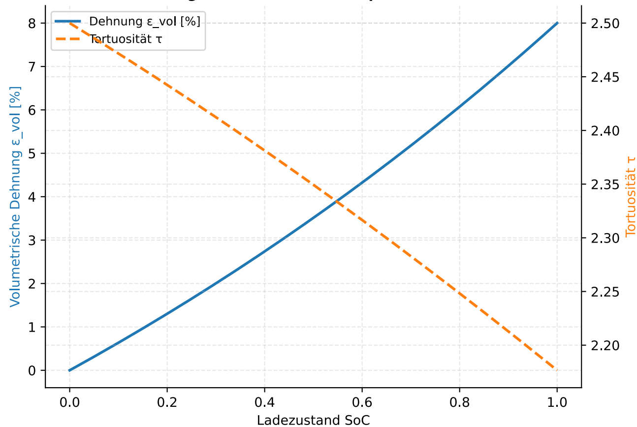
Quellung & Tortuosität des Separators vs. SoC
