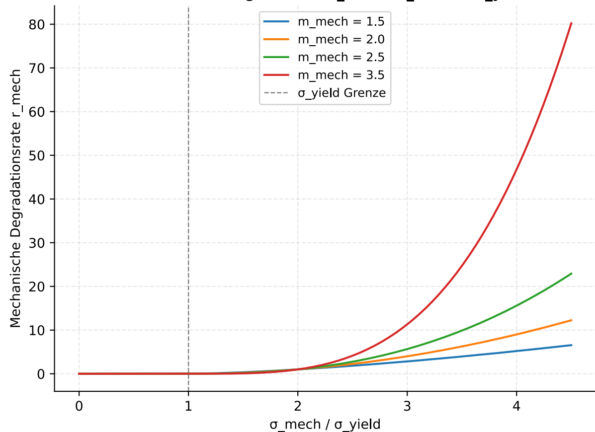
Mechanische Degradation r_{mech}(\sigma_{mech} / \sigma_{yield})
