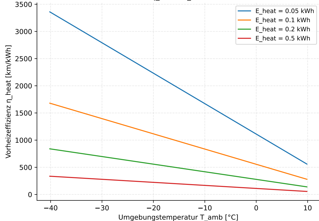
Vorheizeffizienz \eta_{\text{heat}}(T_{\text{amb}}) ( R_0 = 400\text{ km} )
