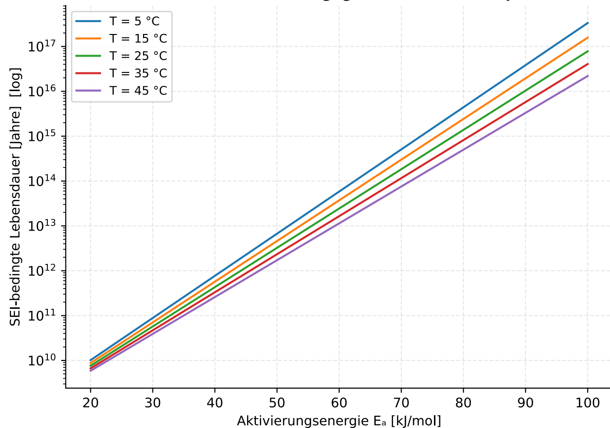
Lebensdauer-Sensitivität gegenüber E_a und Temperatur
