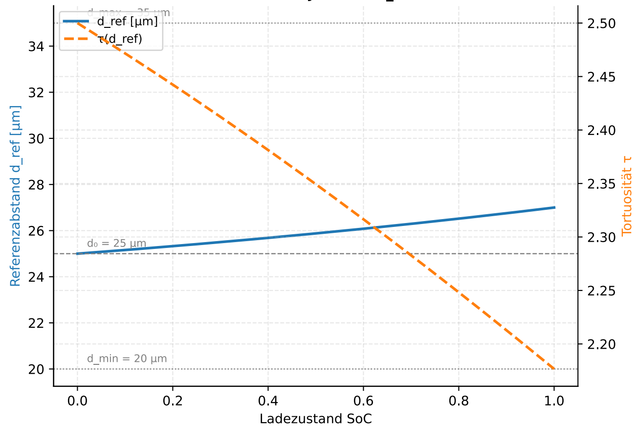
MPC-Referenztrajektorie d_{\text{ref}}(\text{SoC})
