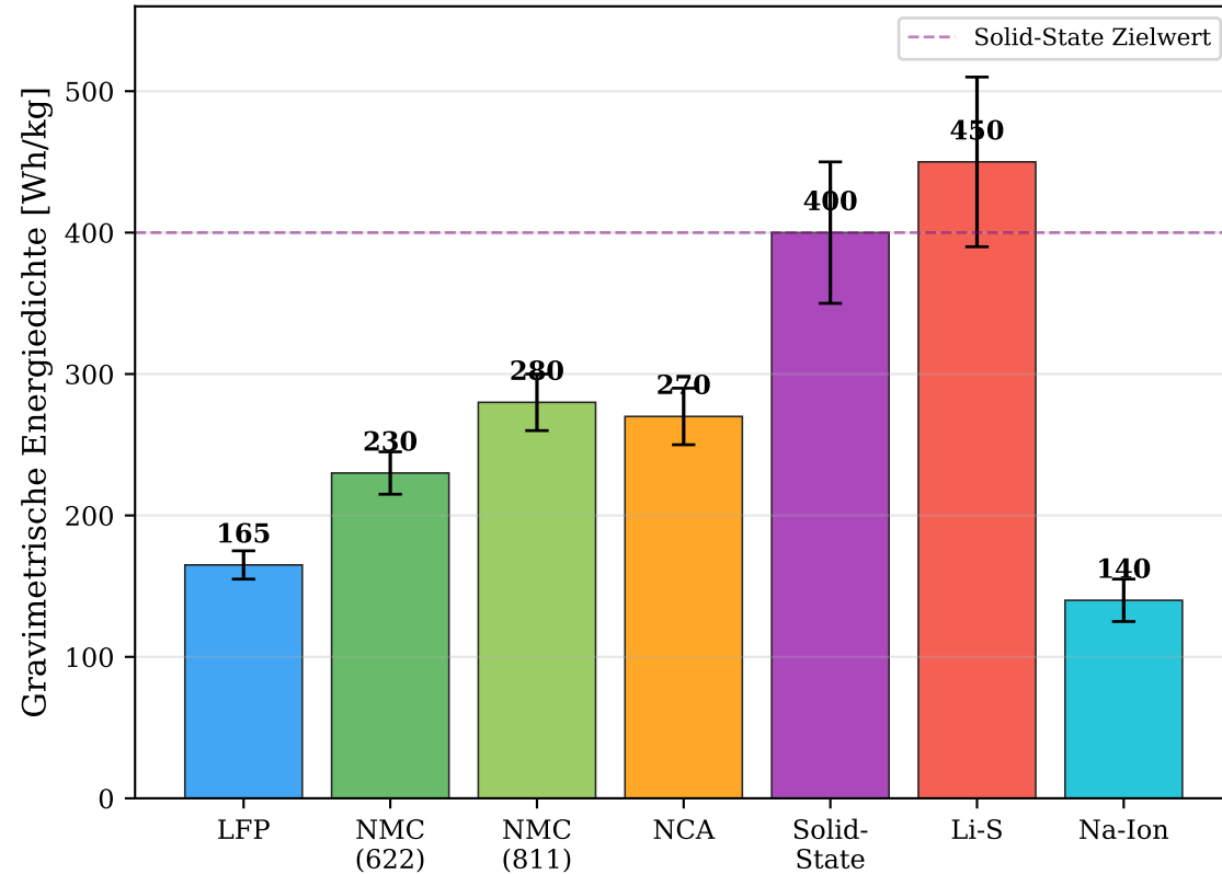
Gravimetrische Energiedichte
