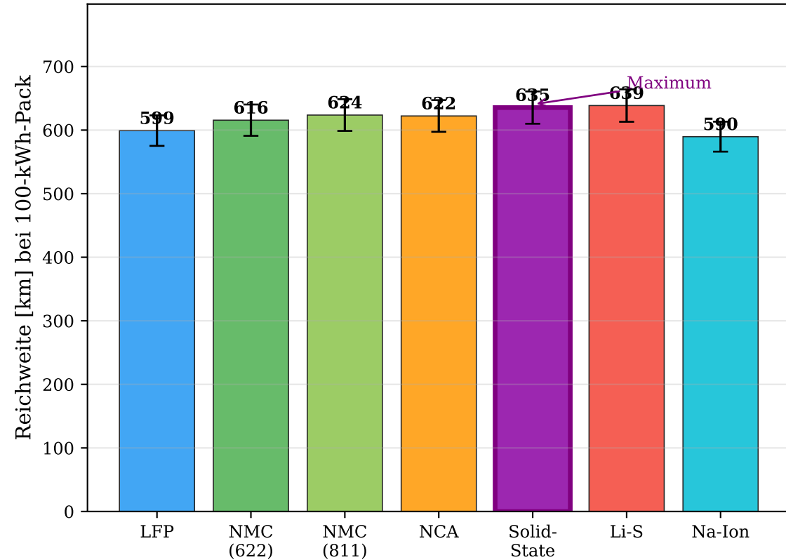
Berechnete Reichweite (Sedan-Klasse, WLTP-Näherung)
