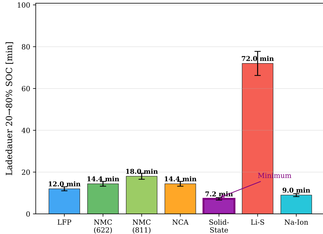
Ladezeit (20→80 % SOC)
