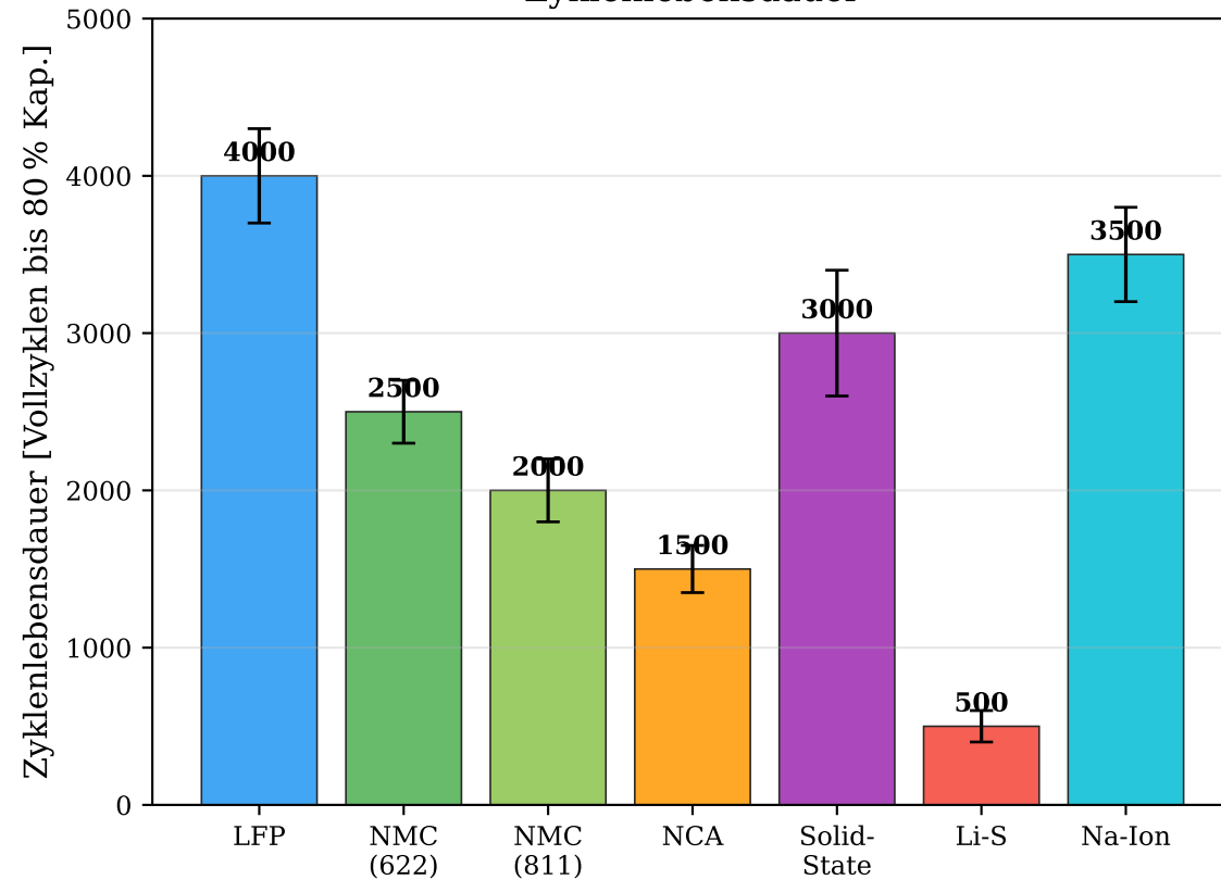
Zyklenlebensdauer
