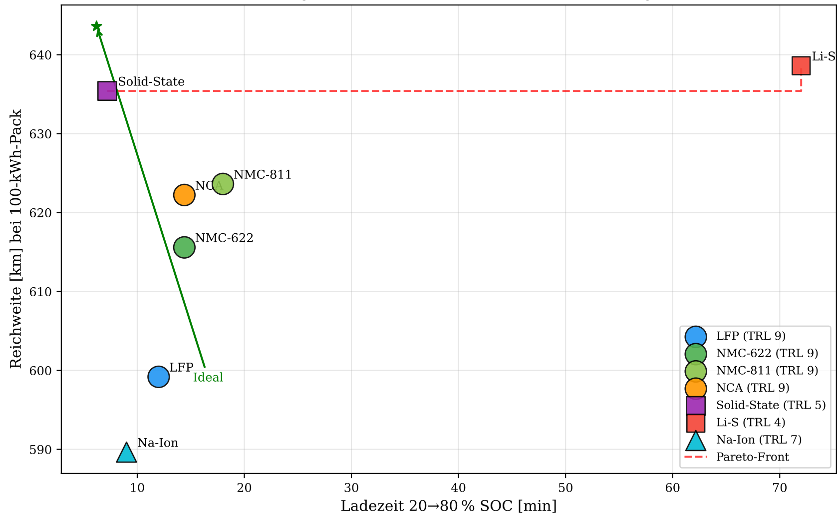
Pareto-Analyse: Reichweite vs. Ladezeit (Markergröße \propto TRL; \circ Serie, \triangle Vorserie, \square Forschung)
