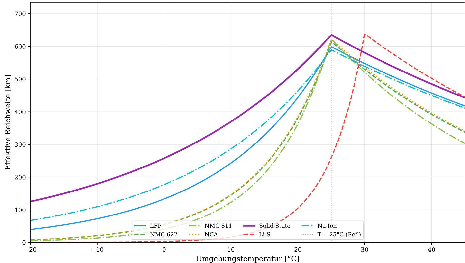
Temperaturabhängige Reichweite (100-kWh-Pack, vereinfachtes Arrhenius-Modell)
