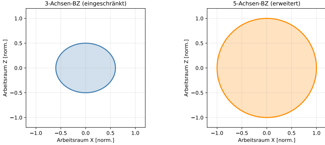
Abbildung 6: Normierter Querschnitt des erreichbaren Arbeitsraums für 3-Achsen- und 5-Achsen-Bearbeitungszentren. Der 5-Achsen-BZ nutzt den vollen Kreis (Normierung auf R = 1 ), während der 3-Achsen-BZ durch eingeschränkte Erreichbarkeit komplexer Geometrien einen kleineren Ellipsoid abdeckt.
