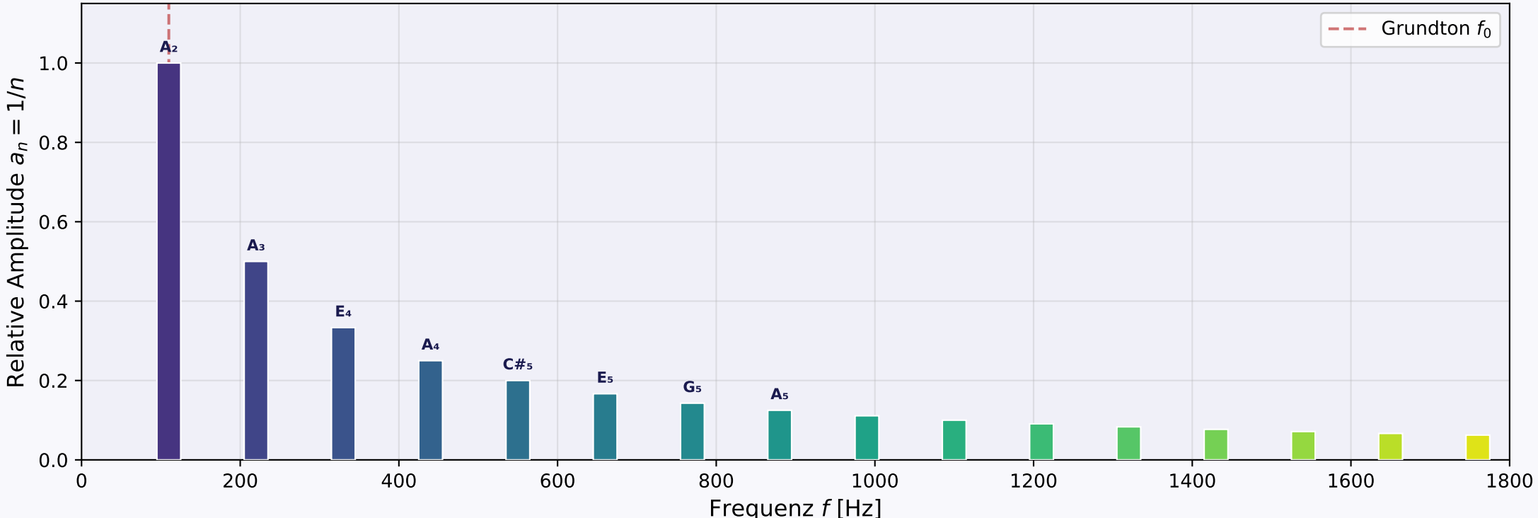
Harmonische Obertonreihe: f_n = n \cdot f_0 , f_0 = 110 \text{ Hz (A}_2)
