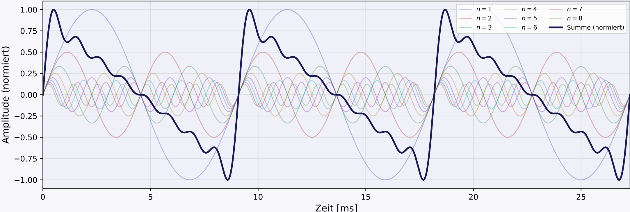
Superposition der ersten 8 Obertöne im Zeitbereich
