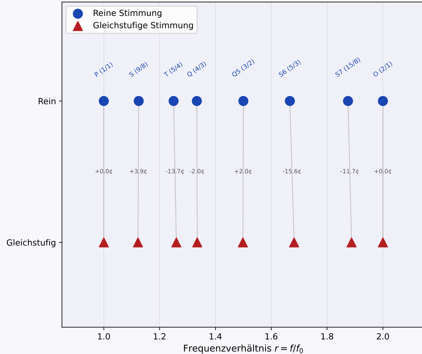
Reine vs. gleichstufige Stimmung (Abweichung in Cent \phi )
