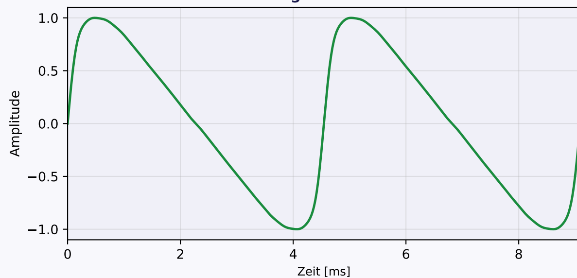
Pfeifenorgel — Zeitbereich
