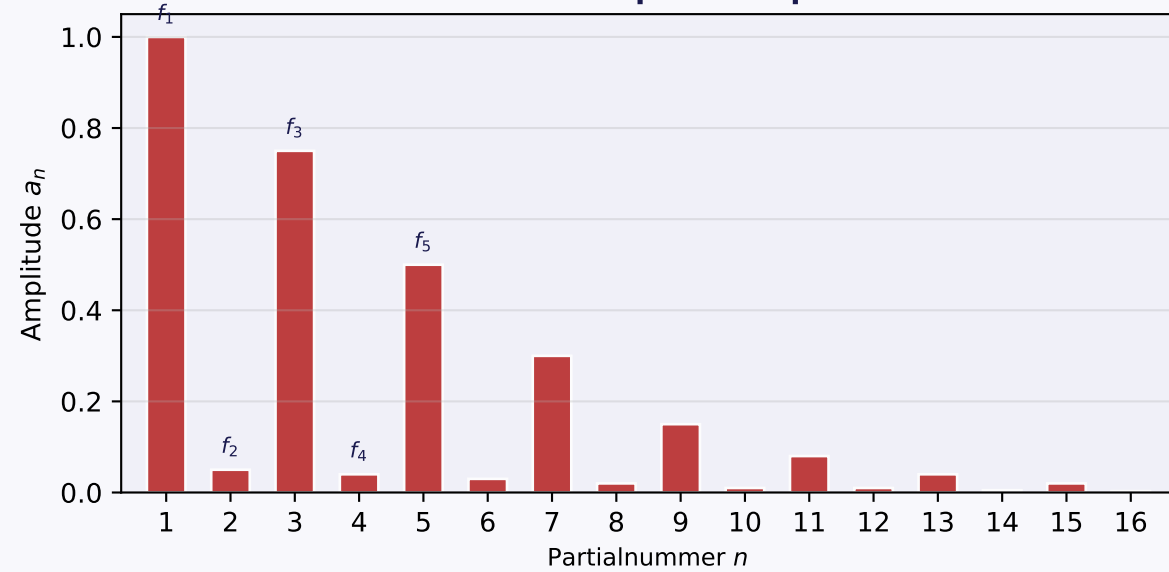
Klarinette — Amplitudenspektrum
