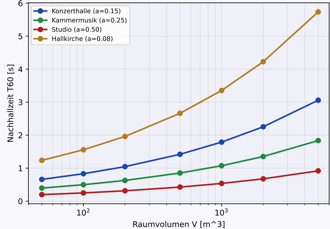
Nachhallzeit nach Sabine: T_{60} = 0.161 V / A
