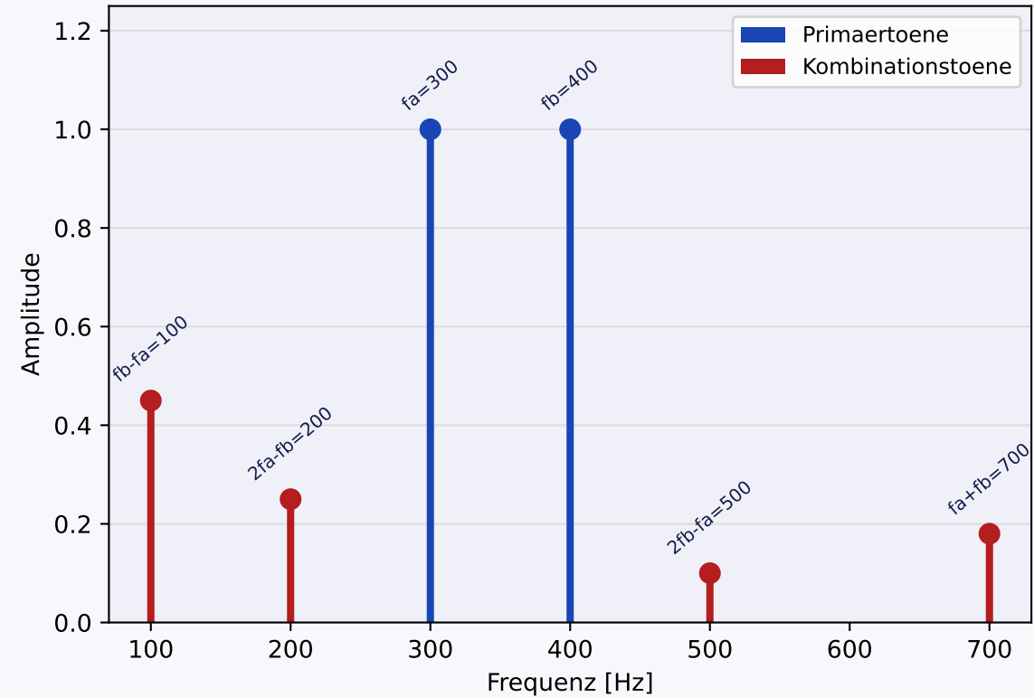
Kombinationstöne bei f_a=300 Hz, f_b=400 Hz
