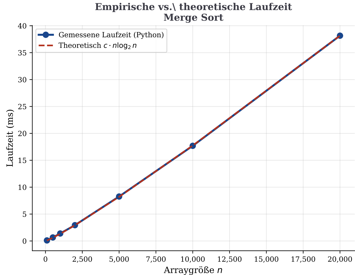
Abbildung 4: Laufzeitanalyse Merge Sort - \mathcal{O}(n \log n)
