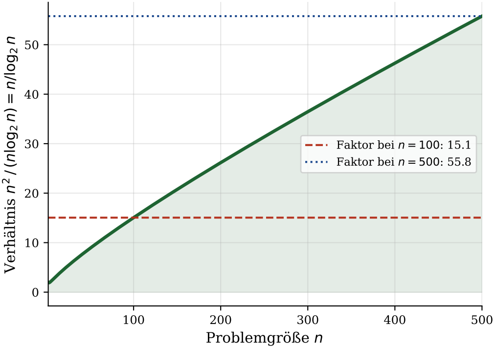
(B) Effizienzgewinn: n^2 vs. n \log n
