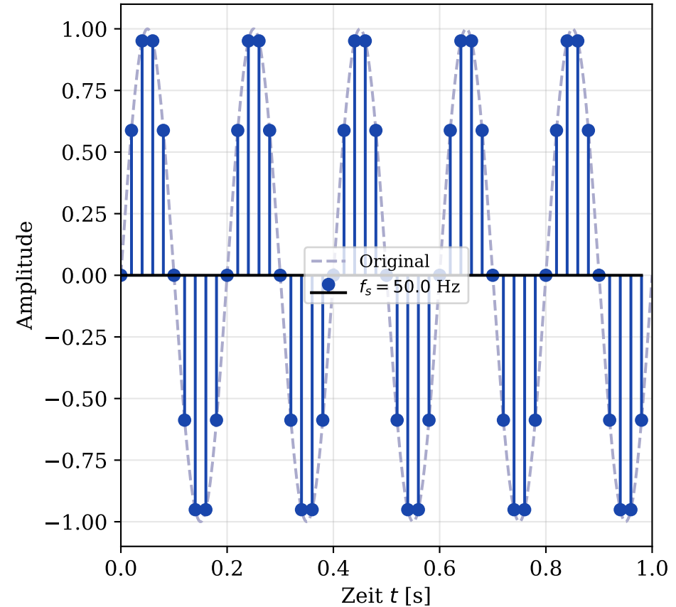
Korrekte Abtastung ( f_s \gg 2f )
