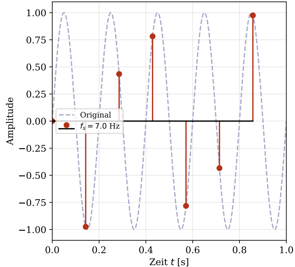
Unterabtastung ( f_s < 2f )
