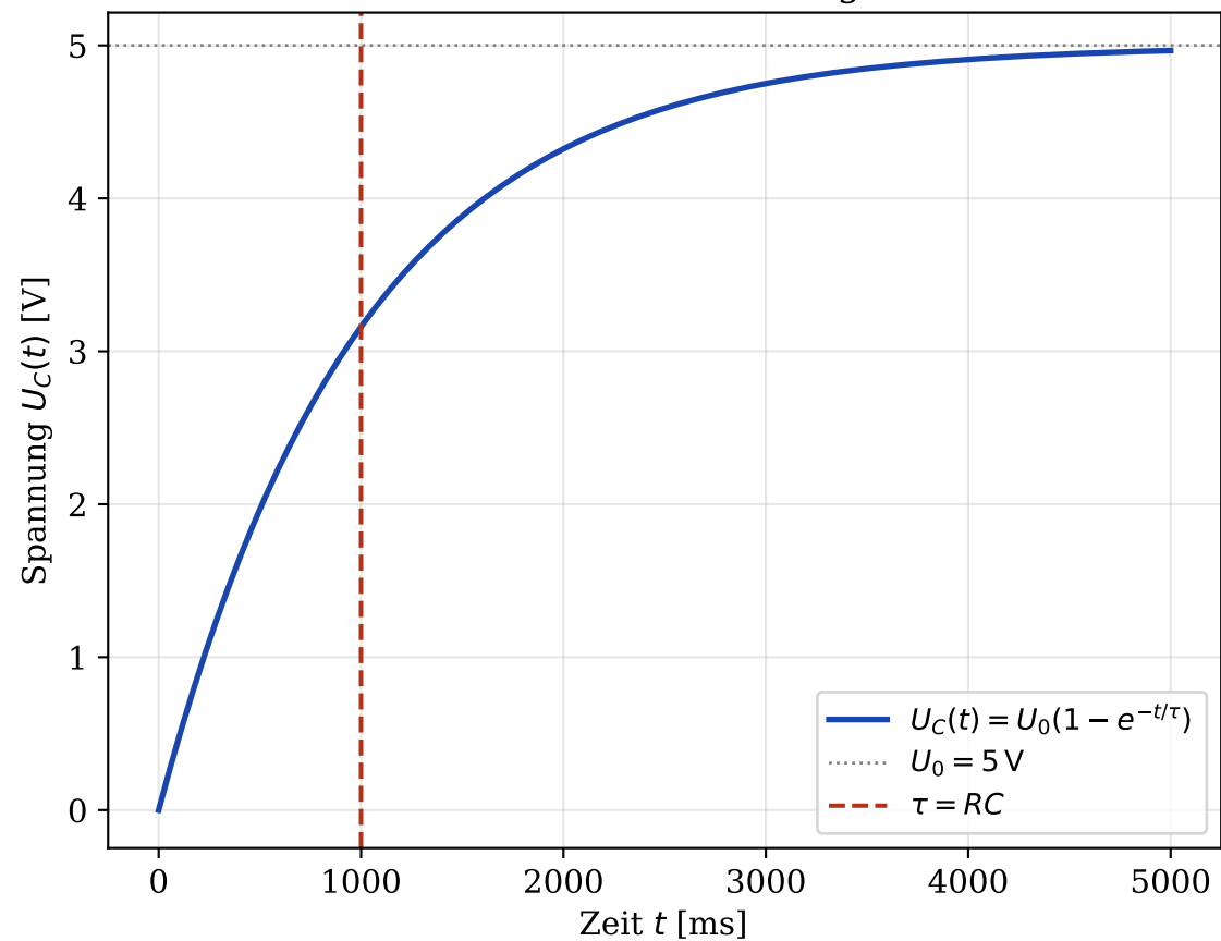
RC-Glied: Aufladung
