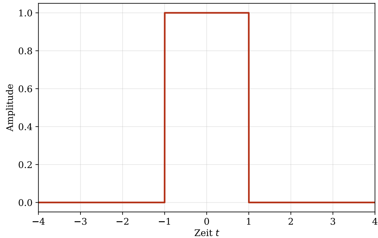
Rechteck-Funktion \Pi(t/T)
