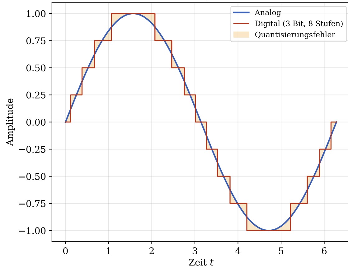
3-Bit-Quantisierung (LSB = 0.2500)
