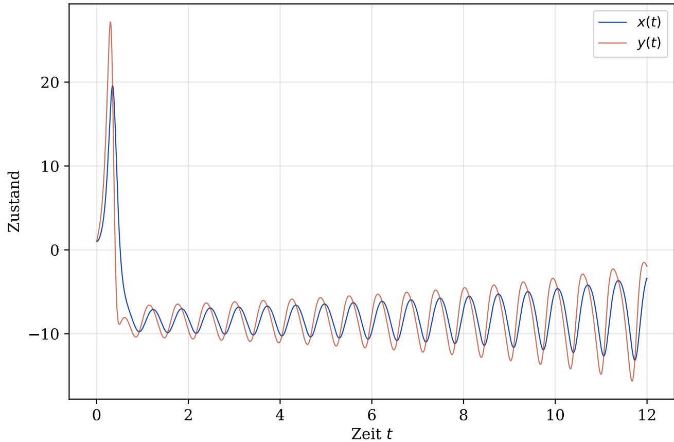
Lorenz: Zeitverlauf
