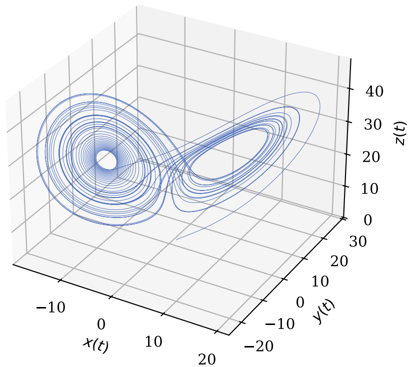
Lorenz-Attraktor (kontinuierlich)
